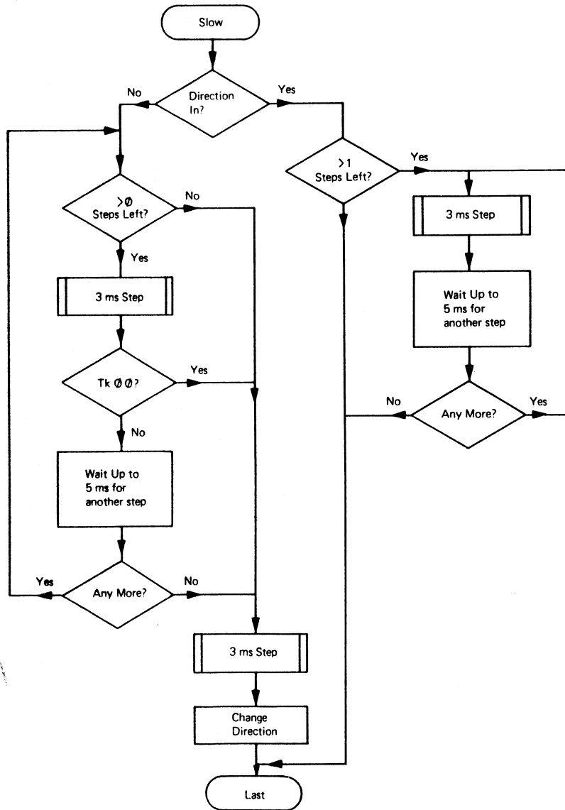
FIGURE 22(d) Step flow chart
